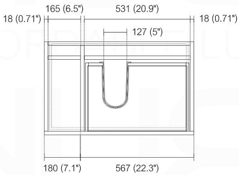
. TOP ELEVATION
